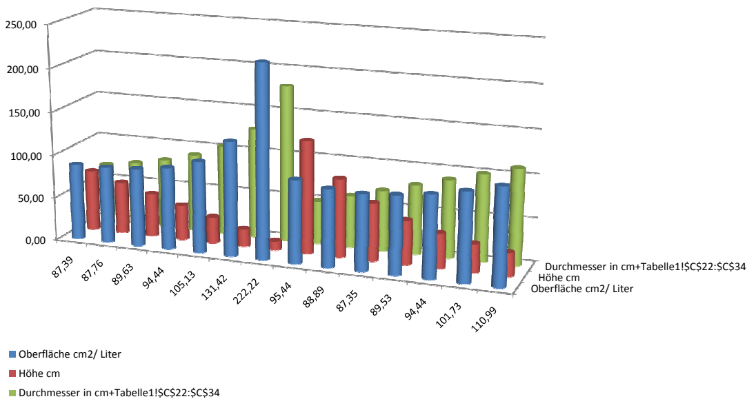
Oberfläche cm2/ Liter in Abhängigkeit von Durchmesser und Höhe bei ca 254 Liter
